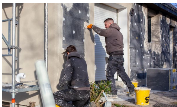
Première couche d'enduit avant mise en place du treillis !
